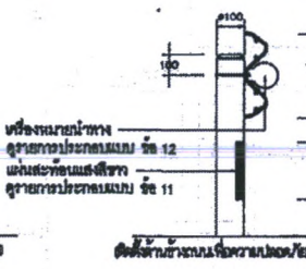
เครื่องหน่วงทาง ดูรายการประกอบแบบ ข้อ 12 แผ่นสะท้อนแสงสีขาว ดูรายการประกอบแบบ ข้อ 11
