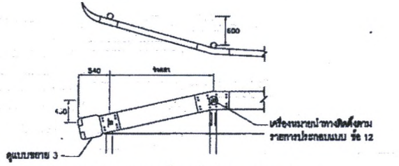
แบบขยาย 1 แสดงการติดตั้งและพื้นปลาย GUARD RAIL มาตราส่วน 1 : 30
