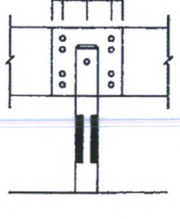
แบบขยาย 2 แสดงการติดตั้งกับแนวสะพานหรือ CONCRETE BARRIER มาตราส่วน 1 : 30
