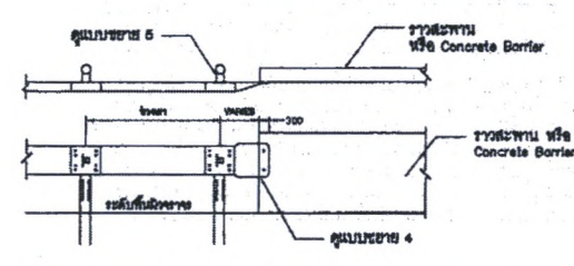
แบบขยาย 2 แสดงการติดตั้งกับแนวสะพานหรือ CONCRETE BARRIER มาตราส่วน 1 : 30
