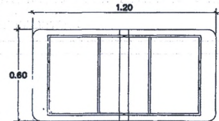
โครงเหล็กถาขนาด 1"x1"x2.3 มม ทาดวยสีกันสนิม เชื่อมโดยรอบ เจาะรูได้นอต 4-๘ มม ขุดสังกะสี
