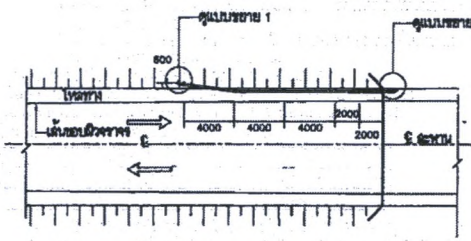
การติดตั้ง GUARD RAIL ตรง มาตราส่วน 1 : 200
