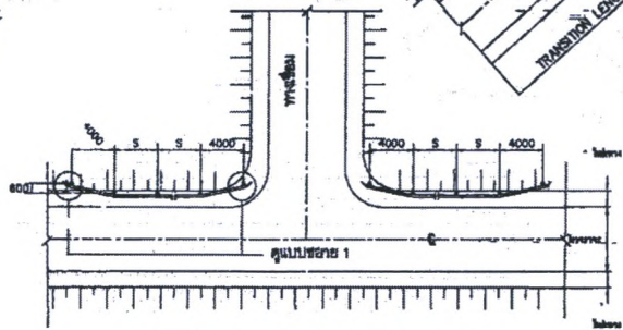
การติดตั้ง GUARD RAIL บริเวณสี่ทางเชื่อม มาตราส่วน 1 : 250
