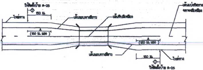
การเดินจราจรในความกว้างสะพานน้อยกว่าความกว้างผิวจราจรถนน ไม่แสดงรายละเอียด
