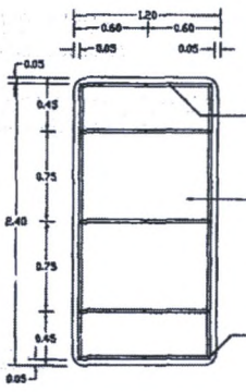
แสดงการติดตั้งป้ายกับโครงเหล็ก ไม่แสดงขนาด
