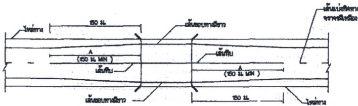
การเดินจราจรในความกว้างสะพานมากกว่าความกว้างผิวจราจรถนน ไม่แสดงรายละเอียด
