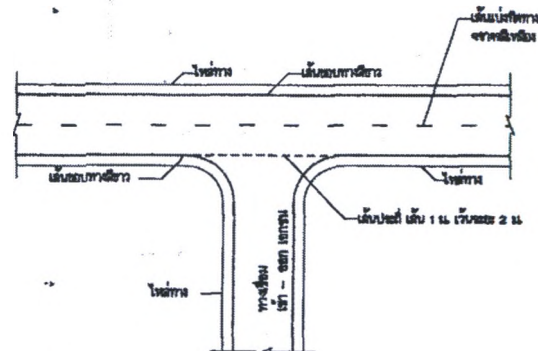
การเดินจราจรทางเชื่อม (ทางเชื่อม เชา - ออก เอกชน)
