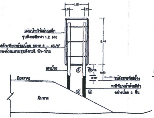
แสดงการติดตั้งป้าย (ด้านหลัง) ไม่แสดงขนาด
