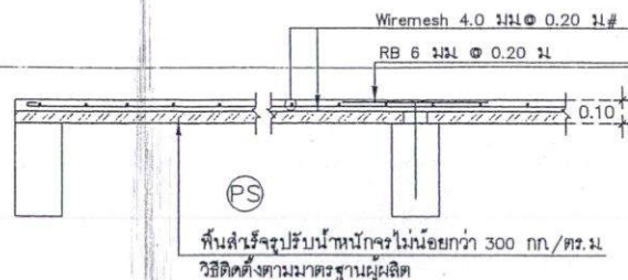
แบบขยายเสริมหลักพิมพ์ 1 : 25
