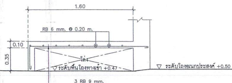
แบบขยายเสริมเหล็กม้านั่ง คสล. 1:25
