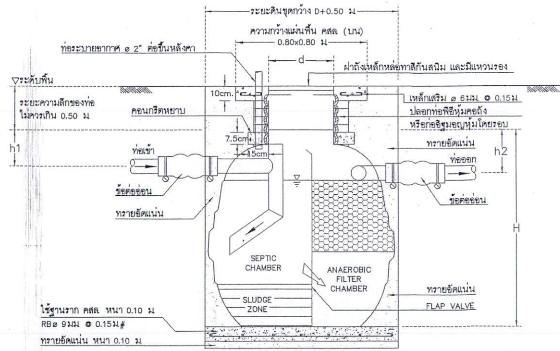
รูปตัดตั้ง
