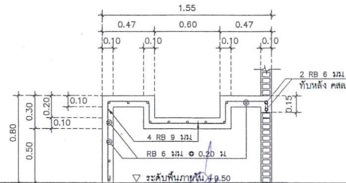
แบบขยายคานาเคอร์ล่างหน้า 1:25
