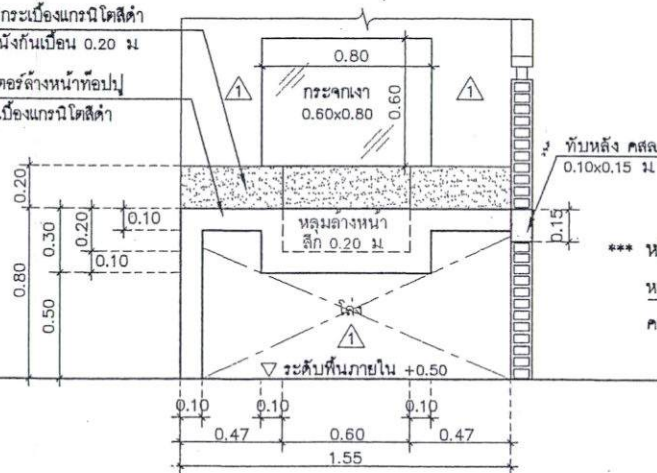
แบบขยายรูปด้านหน้าคานาเคอร์ล่างหน้า 1:25
