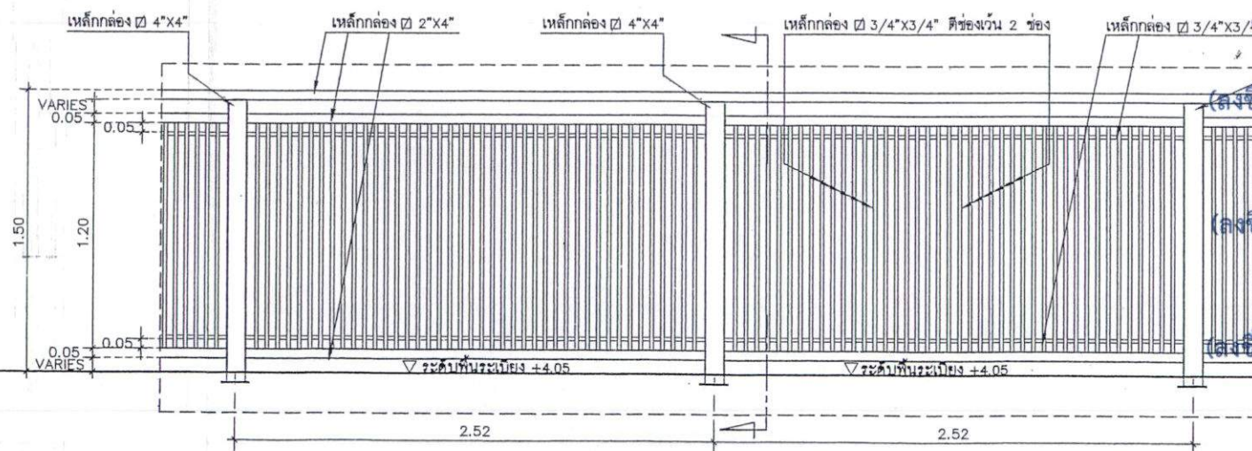
แบบขยายรูปด้านหน้าคานาเคอร์ล่างหน้า 1:25
