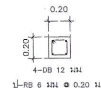
CX1 (0.20x0.20) (เสาฐานล่าง รับฐานพักบันได)
