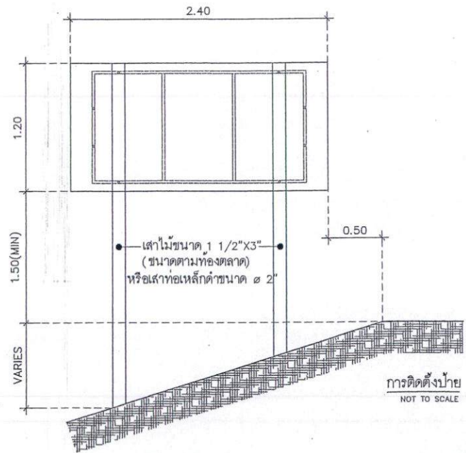
รายละเอียดด้านหน้าป้ายประชาสัมพันธ์โครงการ NOT TO SCALE
