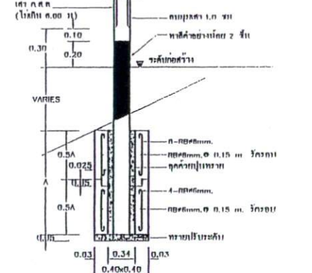
แสดงการปักเสาป้ายโครงการ ไม่แสดงมาตราส่วน
