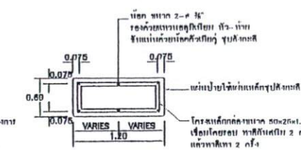
รายละเอียดด้านหลังป้ายโครงการ ไม่แสดงมาตราส่วน
