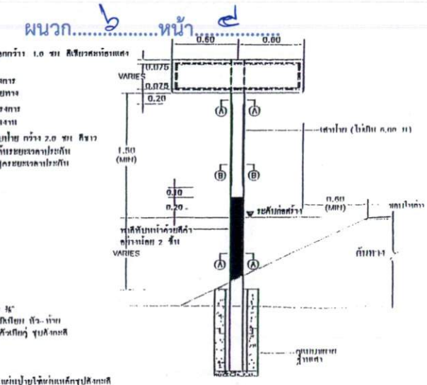
แสดงการปักเสาป้ายโครงการ ไม่แสดงมาตราส่วน
