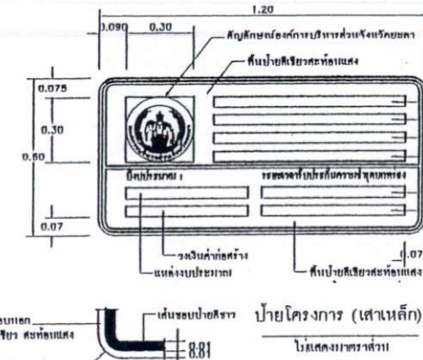
ป้ายโครงการ (เสาเหล็ก) ไม่แสดงมาตราส่วน
