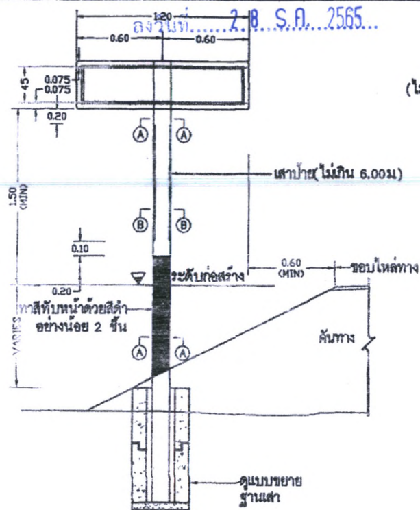
แสดงการปักเสาป้าย (ข้อที่ปลดออก) และ (น-1)
