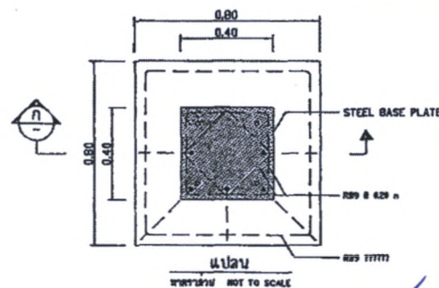
รายละเอียดป้าย
