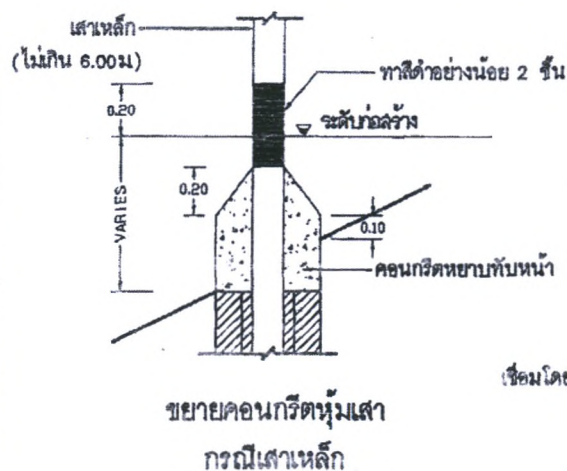
แสดงการปักเสาป้าย (ข้อที่ปลดออก) และ (น-1)
