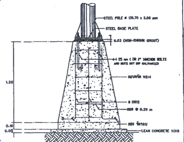
รูปตัด ๑ ก รายละเอียดฐานเสา MAST ARM
