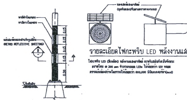
รายละเอียดการติดตั้งป้าย
