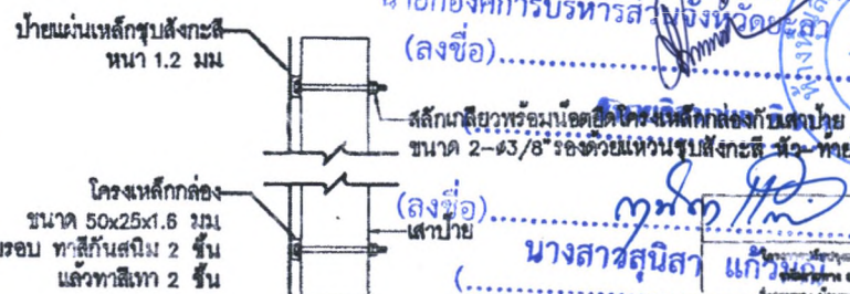
แสดงการติดตั้งโครงเหล็กกล่องกับเสาป้าย
