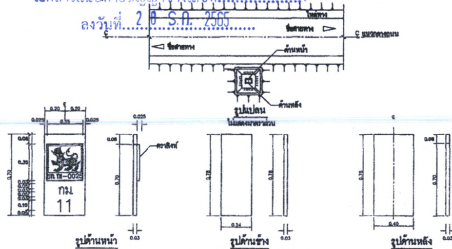
แสดงรายละเอียดแนบปูนสำเร็จรูป
