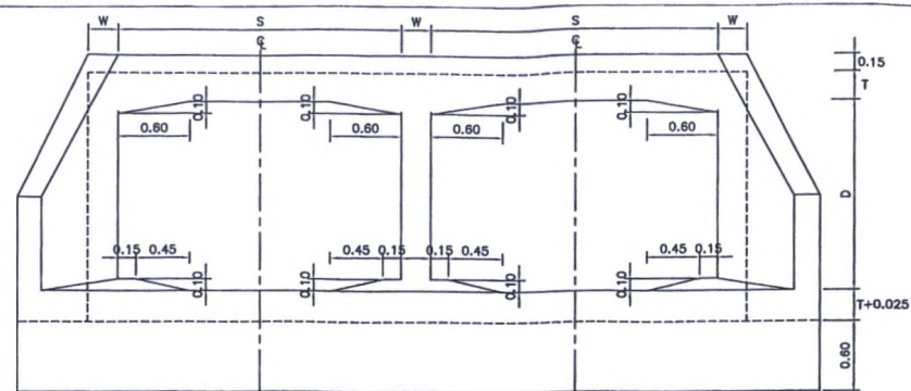
รูปด้านหน้า มาตราส่วน 1:2
