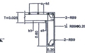
BOTTOM BEAM รายละเอียด (2) มาตราส่วน 1:20 (-)
