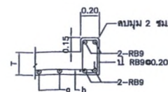
TOP BEAM รายละเอียด (1) มาตราส่วน 1:20
