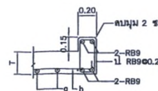
TOP BEAM รายละเอียด (1) มาตราส่วน 1:20 (-)
