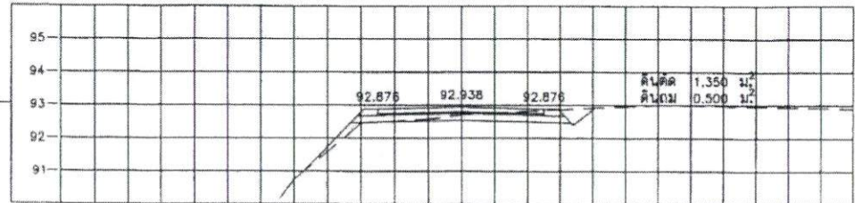
STA. 0+625.000 NGL = 92.696
