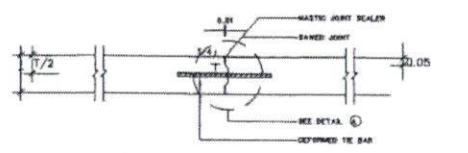
LONGITUDINAL JOINT
