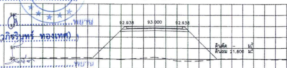
STA. 0+350.000 NGL = 90.176
