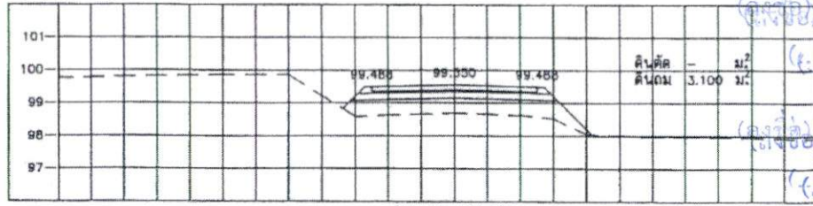
STA. 0+025.000 NGL = 98.693
