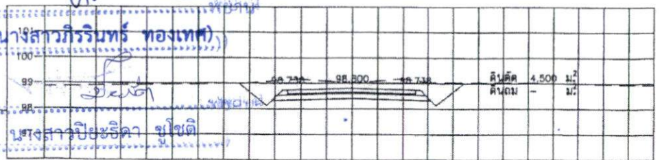
STA. 0+125.000 NGL = 99.000
