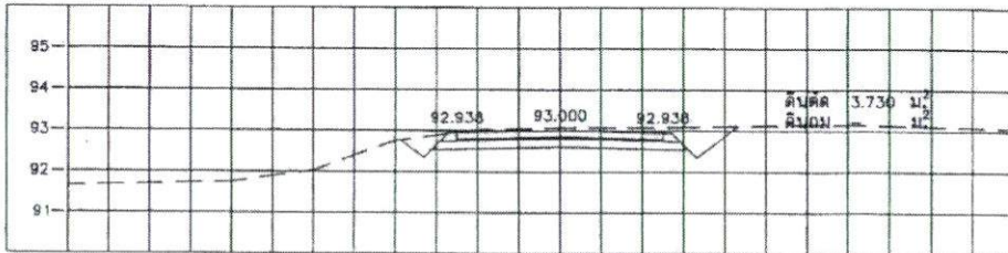
STA. 0+525.000 NGL = 93.066
