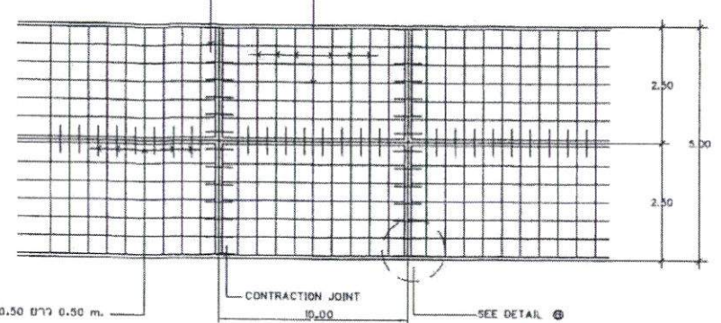
แปลนแลคกวางเสริมเหล็กถนน ค.ล.ล.
