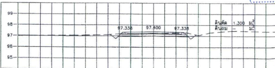
STA. 0+225.000 NGL = 96.790
