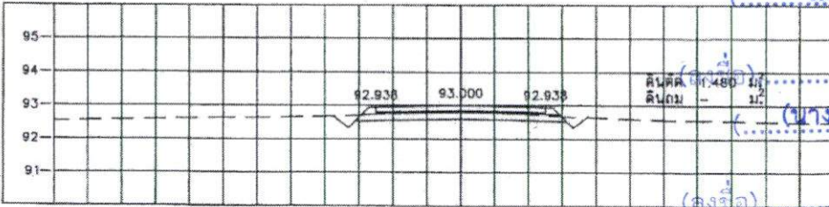
STA. 0+475.000 NGL = 92.851
