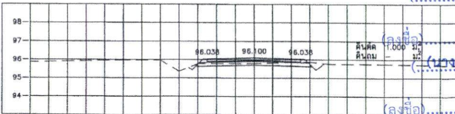
STA. 0+250.000 NGL = 95.790
