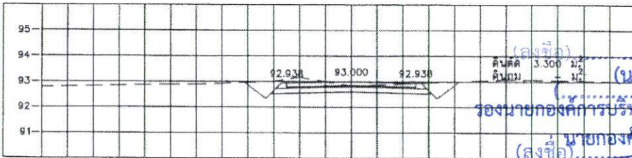
STA. 0+500.000 NGL = 92.828
