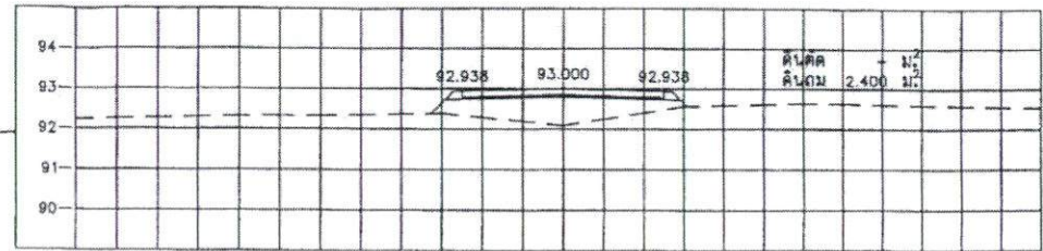
STA. 0+425.000 NGL = 92.088
