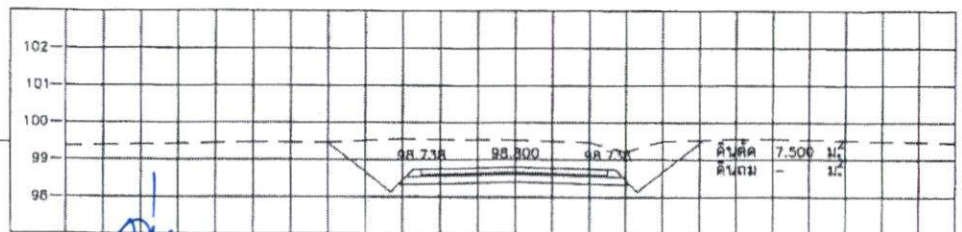
STA. 0+175.000 NGL = 99.520
