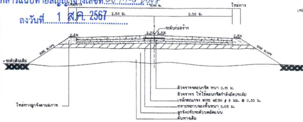
รูปตัดแนวดิ่ง โครงสร้างถนนคอนกรีตเสริมเหล็กและคูน้ำบดอัดผิว
