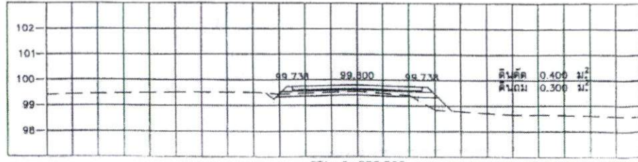
STA. 0+000.000 NGL = 99.540
