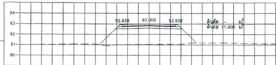
STA. 0+400.000 NGL = 91.050
