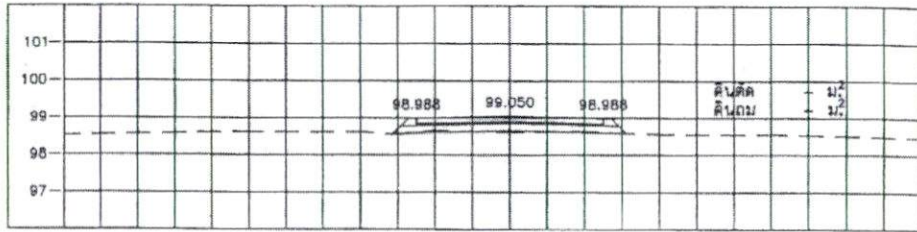
STA. 0+075.000 NGL = 98.610
