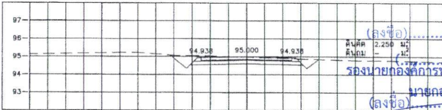
STA. 0+275.000 NGL = 94.980
