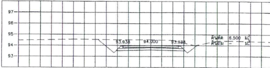
STA. 0+300.000 NGL = 94.522
