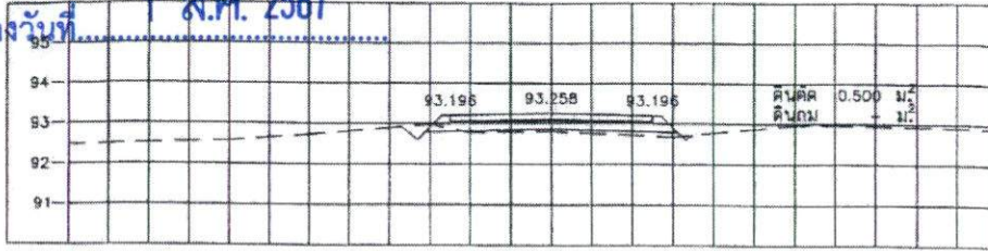
STA. 0+325.000 NGL = 92.790
