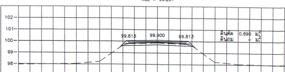
STA. 0+000.000 NGL = 99.857
