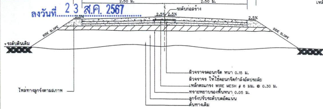
รูปตัดแนวดิ่ง โครงสร้างถนนคอนกรีตเสริมเหล็กและคุณสมบัติวัสดุ
