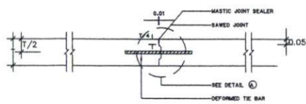
LONGITUDINAL JOINT
