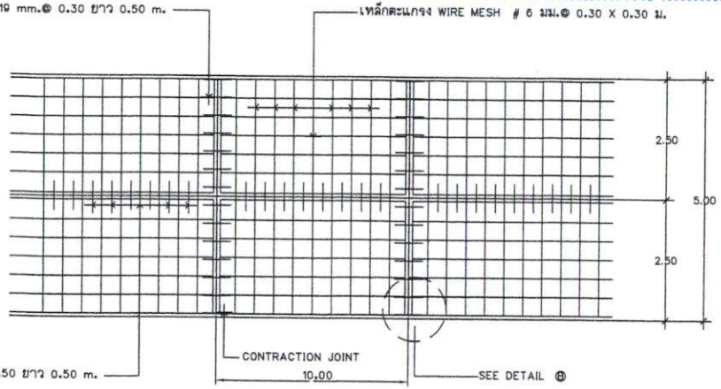
แปลนแสดงการเสริมเหล็กถนน ค.ล.ด.
