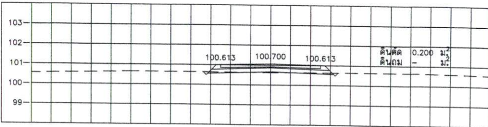
STA. 0+300.000 NGL = 100.625
