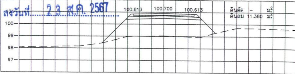
STA. 0+100.000 NGL = 99.043
