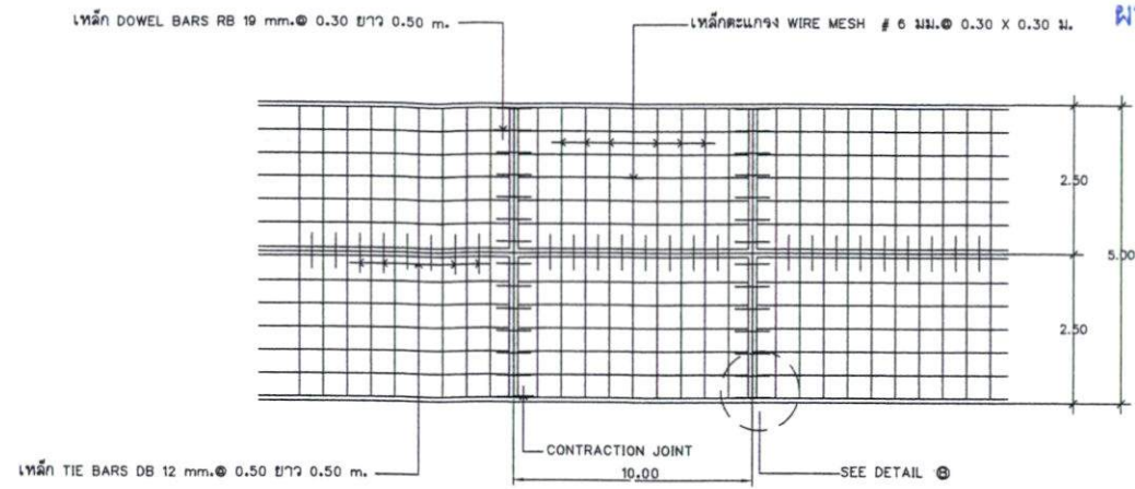
แบบนแสดงการเสริมเหล็กถนน ค.ล.ค.
