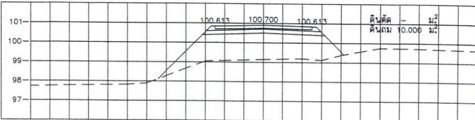
STA. 0+075.000 NGL = 99.143
