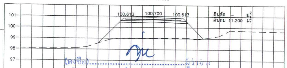
STA. 0+200.000 NGL = 99.038
