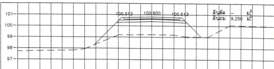
STA. 0+050.000 NGL = 99.231
