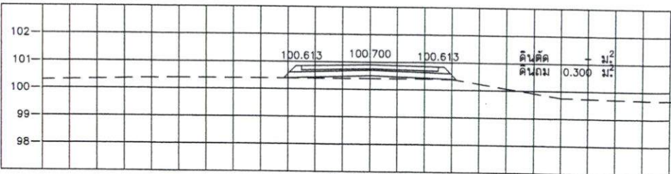
STA. 0+250.000 NGL = 100.393
