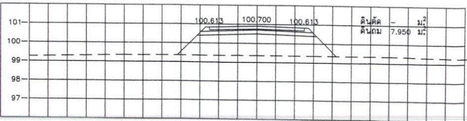
STA. 0+225.000 NGL = 99.361
