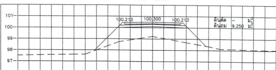
STA. 0+025.000 NGL = 99.231
