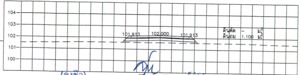
(ลงชื่อ)..... STA. 0+400.000 NGL = 101.586
