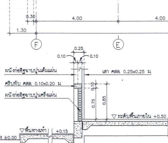
แบบขยายรูปตัด ① ก่อผนังอิฐชั้นที่ 1 1 : 50
