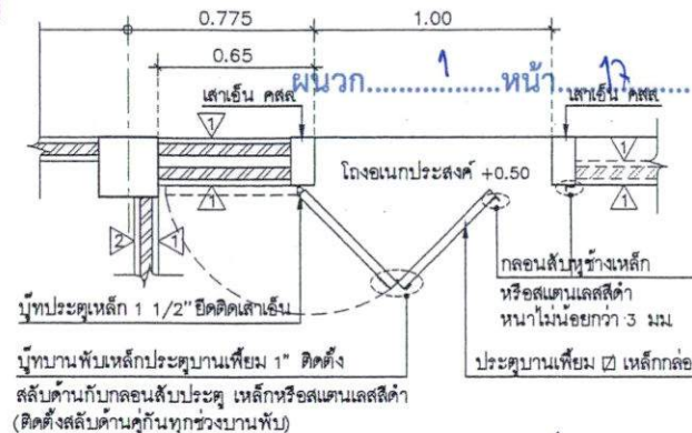
แบบขยายแปลน D2 1:25 ทิศทางการมองดูบาน
