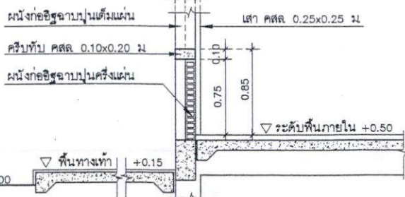
แบบขยายรูปตัด 1 ก่อผนังอิฐขึ้นที่ 1 1 : 50
