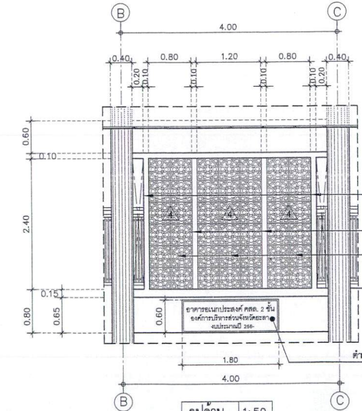
รูปด้าน 1:50
