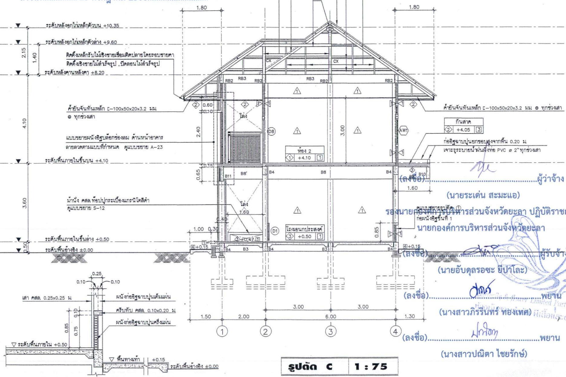
แบบขยายรูปตัด ① ก่อผนังอิฐชั้นที่ 1 1 : 50
