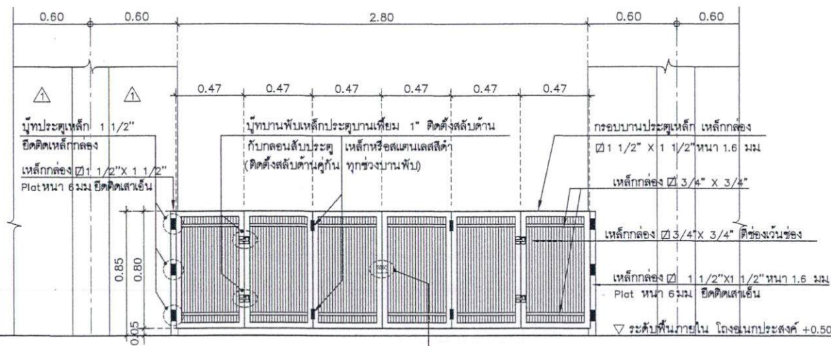
แบบขยายรูปด้าน D1 1:25 ทิศทางการมองดูบาน
