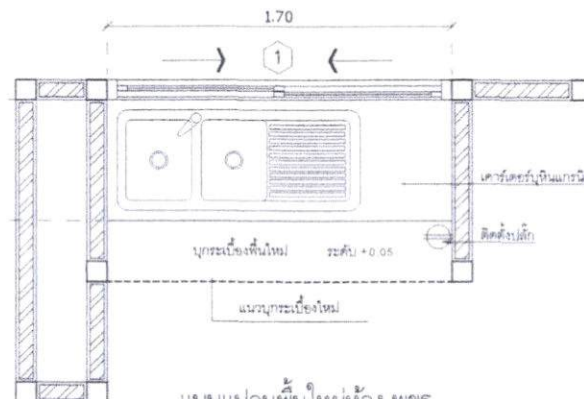
แบบแปลนพื้นใหม่ห้อง พชร. SCALE 1:25
