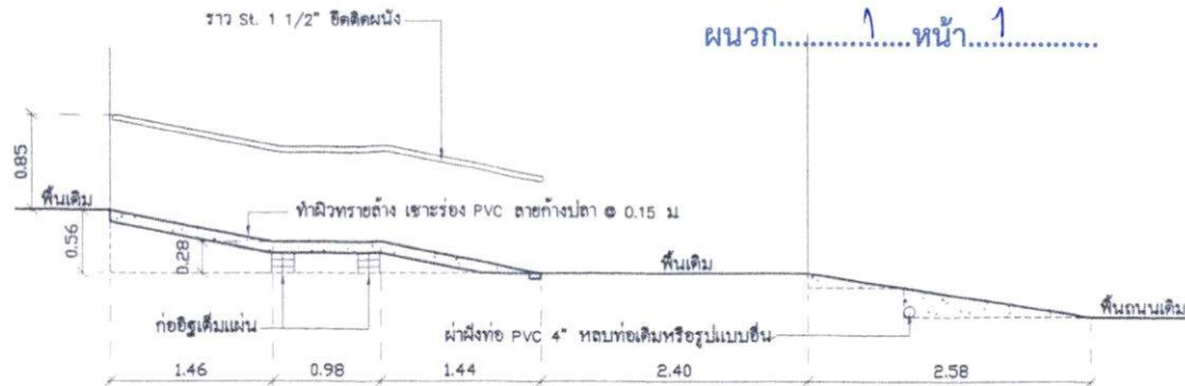
รูปด้านตัดปรับปรุงทางลาดคนพิการ SCALE 1 : 50
