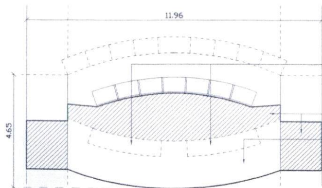
แบบแปลนพื้นเดิมห้อง พชร. SCALE 1:25
