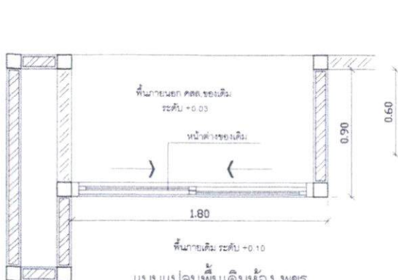
แบบแปลนพื้นเดิมห้อง พชร. SCALE 1:25
