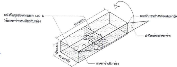
ก่อดองลาดตาข่ายแบบ Gabion
