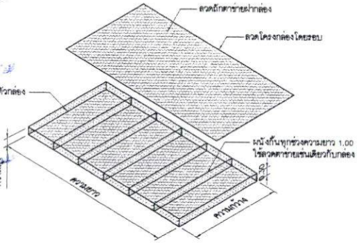
ก่อดองลาดตาข่ายแบบ Mattress
