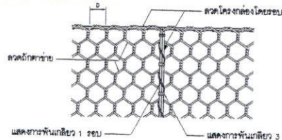
รูป "H" แสดงการมัดลวดตาข่าย
