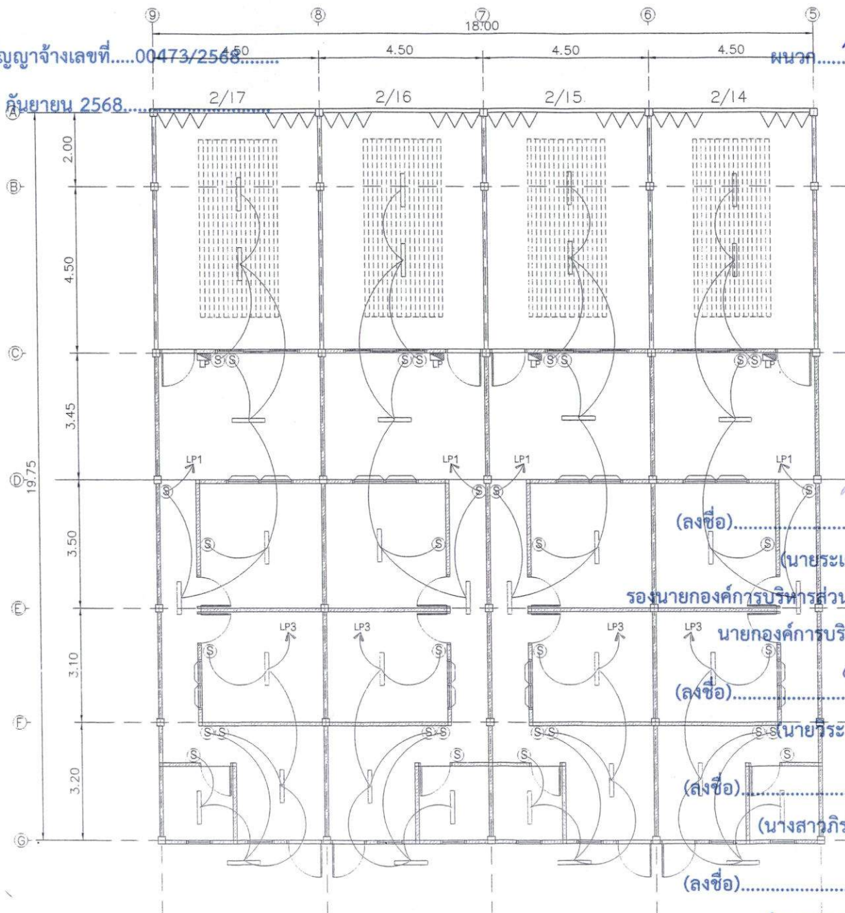
แบบผังโคมไฟส่องสว่าง Scale 1:100
