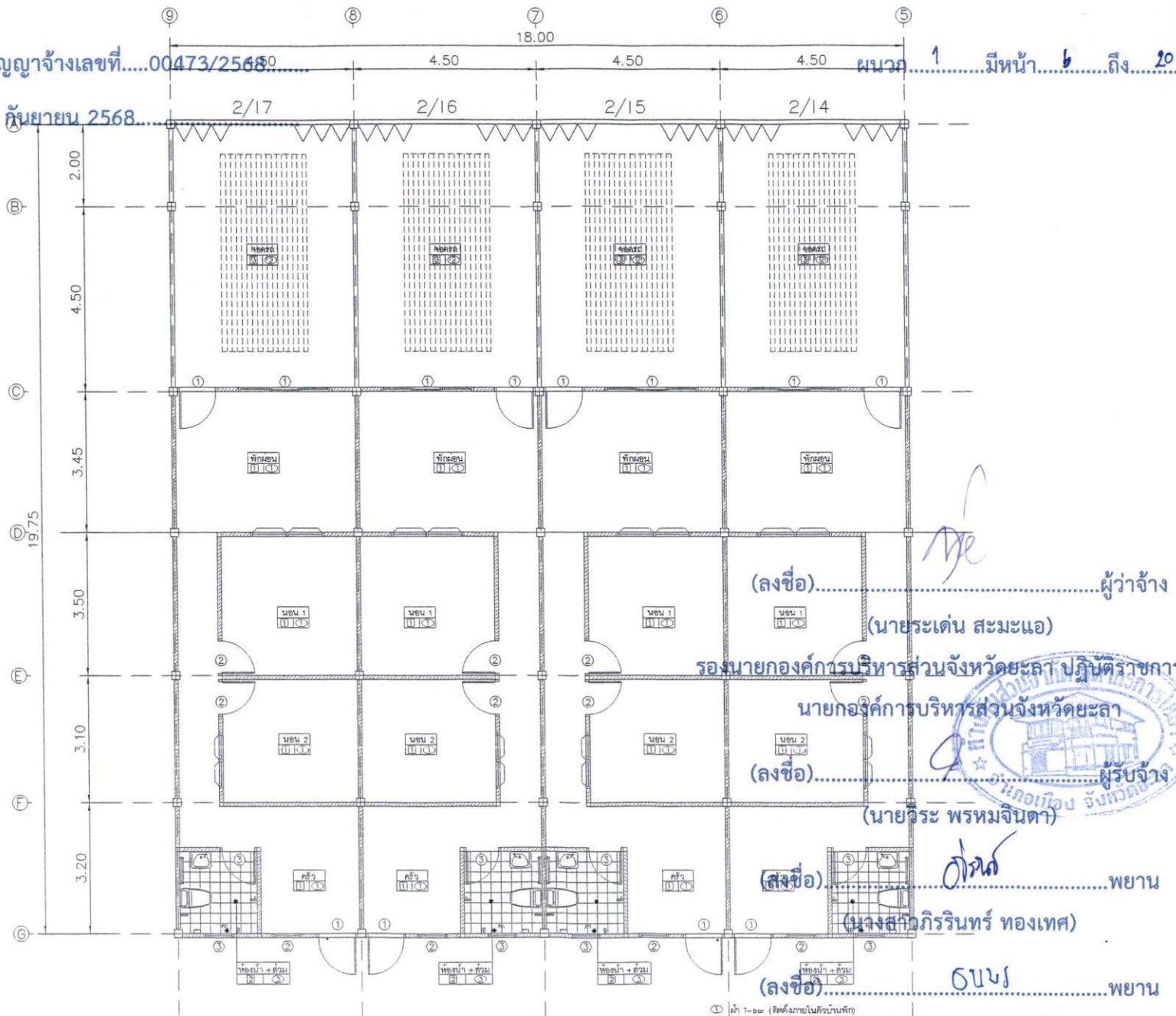
แบบแปลนพื้นอาคาร Scale 1:100 บ้านพักข้าราชการบริเวณถนนเอกราช
