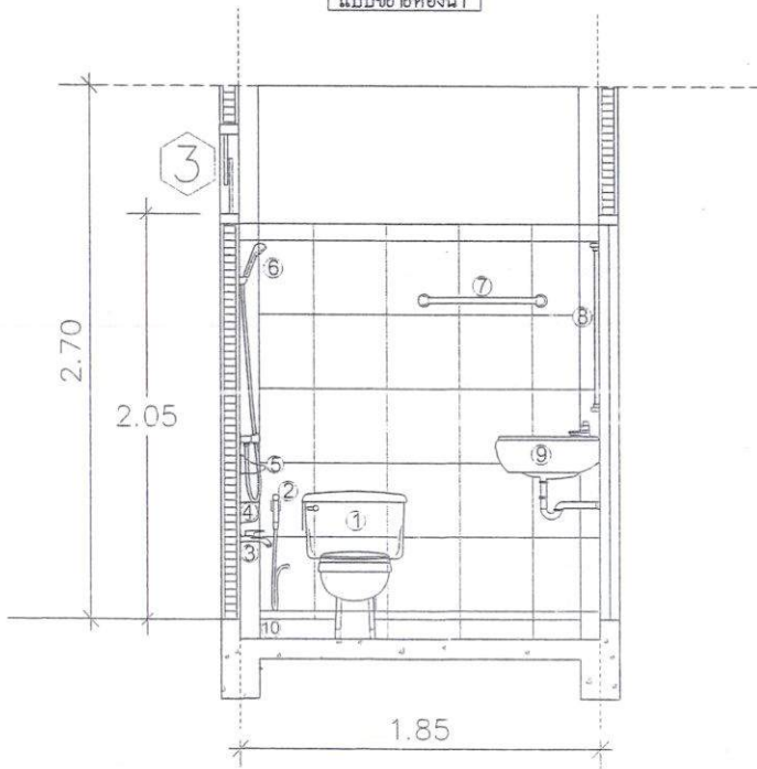
รูปตัด A Scale 1:100 แบบขยายห้องน้ำ
