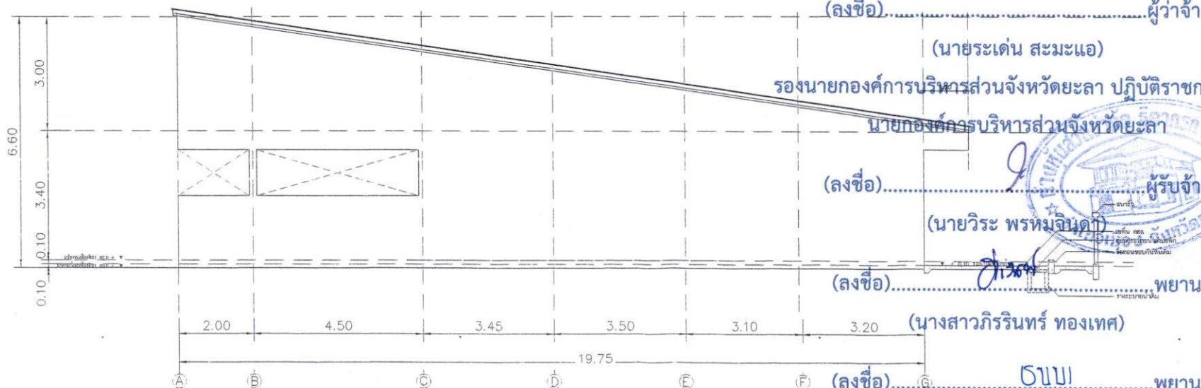
รูปคานขวา Scale 1:100 บ้านพักเรือนแถว 11 คูหา
