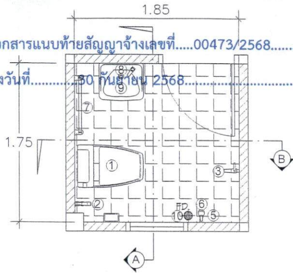
แปลน Scale 1:100 แบบขยายห้องน้ำ
