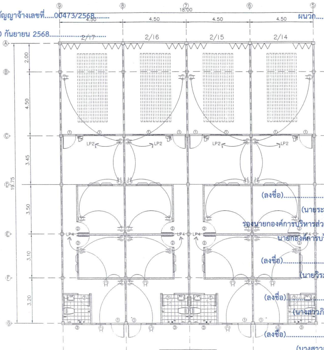
แบบแปลน เตารับไฟฟ้า Scale 1:100
