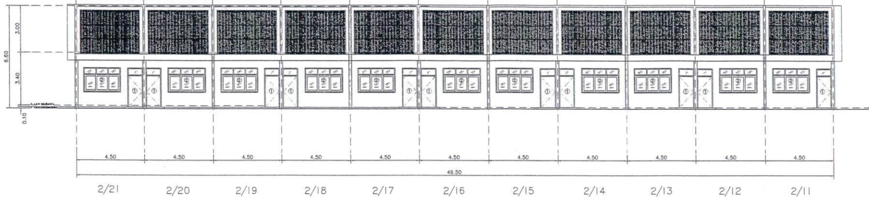
รูปด้านหน้า Scale 1:175 บ้านพักเรือนแถว 11 ตูหา
