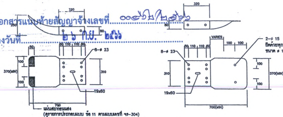
แบบขยาย 3 แผ่นปลาย - GUARD RAIL มาตราส่วน 1 : 10
