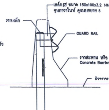
แบบขยาย 5 มาตรา 11 1 : 10
