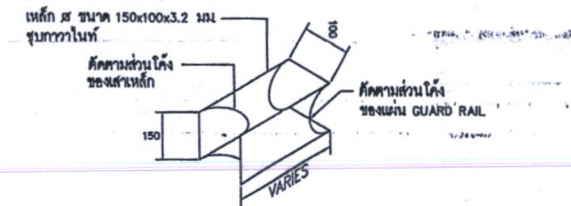
แบบขยาย 6 เหล็กกล่องสำหรับปรับระยะ ไม่ถอดรื้อ
