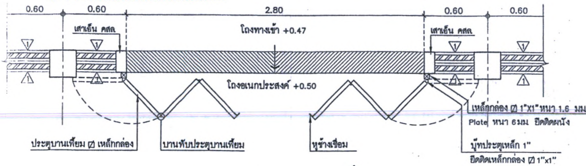
แบบขยายแปลน D1 มาตรฐาน 1:25
