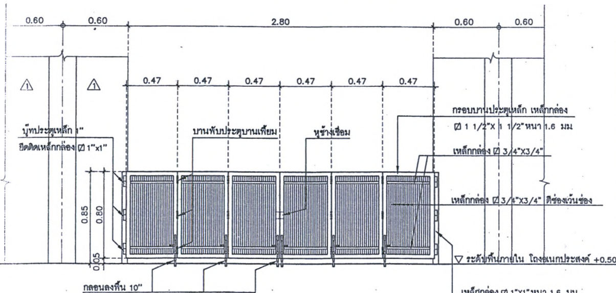
แบบขยายรูปด้าน D1 มาตรฐาน 1:25
