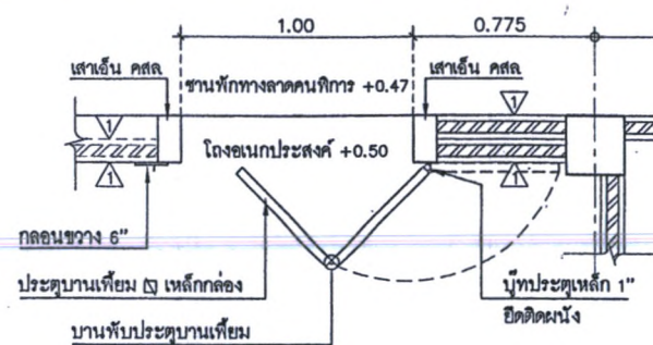
แบบขยายแปลน D2 มาตรฐาน 1:25
