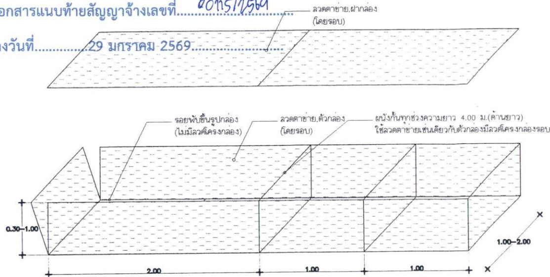
รูปที่ 1 รูปกล่อง GABION & MATTRESS 1:50
