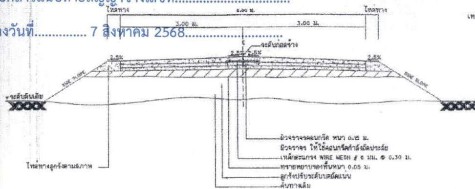
รูปตัดแสดงโครงร่างถนนคอนกรีตเสริมเหล็กและคูน้ำบดอัด
