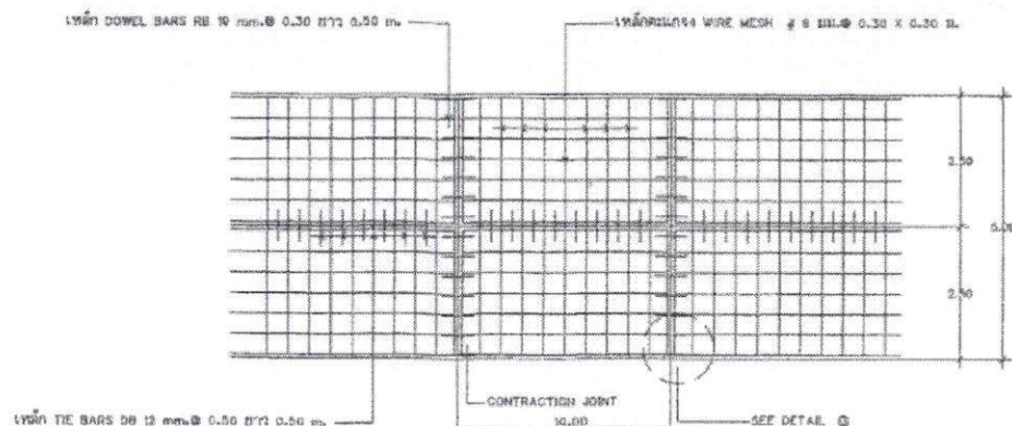
แบบฉบับแสดงการเสริมเหล็กถนน ค.จ.ค.
