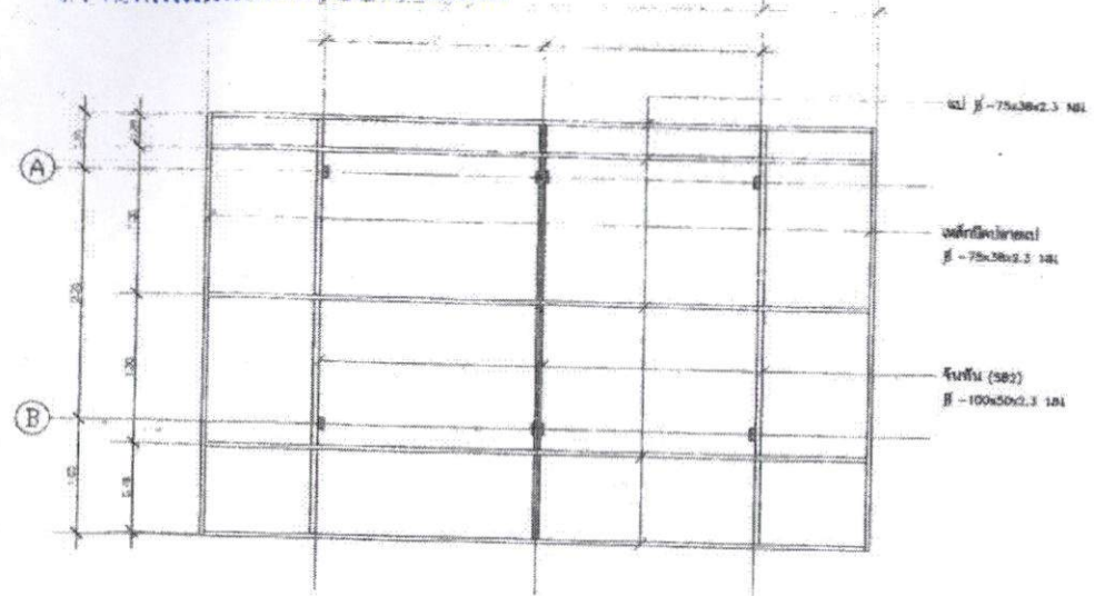
แบบผังโครงสร้าง SCALE 1:50
