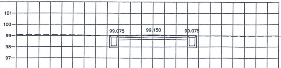
STA. 0+000.000 NGL = 99.148
