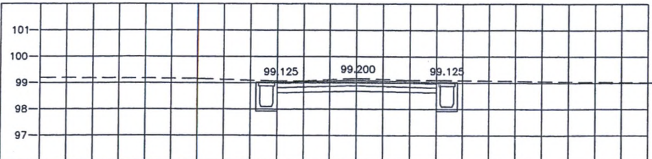
STA. 0+025.000 NGL = 99.215
