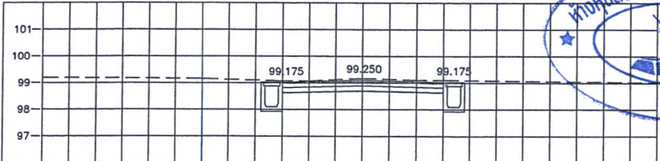
STA. 0+050.000 NGL = 99.317
