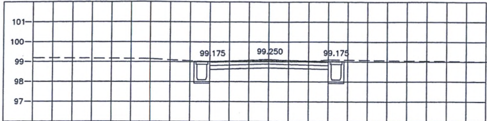
STA. 0+075.000 NGL = 99.230
