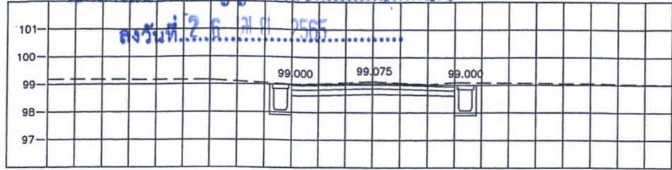
STA. 0+100.000 NGL = 99.047
