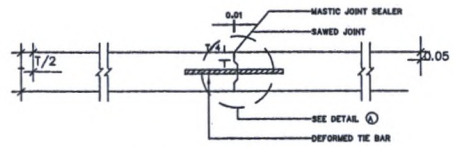
LONGITUDINAL JOINT
