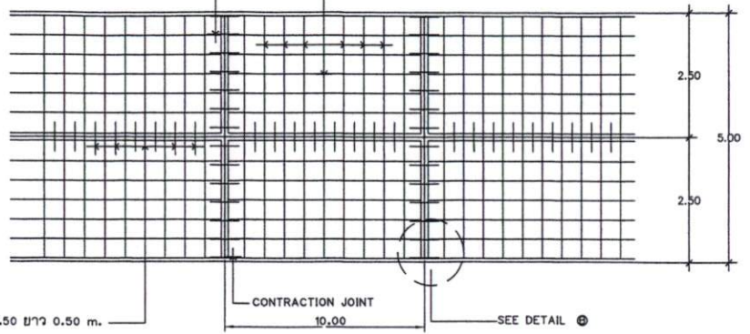
แปลนแฉ่งการเสริมเหล็กถนน ค.ล.ล.
