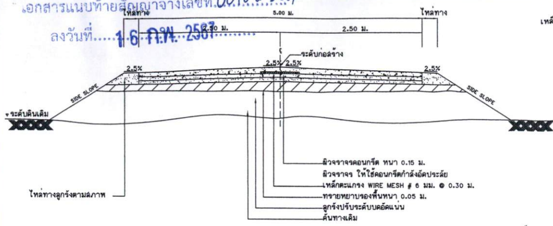
รูปตัดแฉ่งโครงสร้างถนนคอนกรีตเสริมเหล็กและคุณลุ่มบิตูวัลดู
