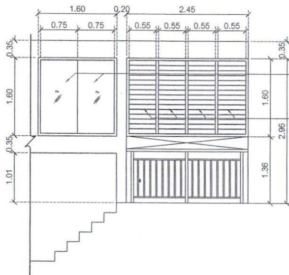
รูปด้านหน้า 1 : 50
