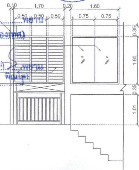
รูปด้านหน้า 1 : 50
