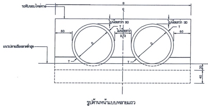
ตารางแสดงขนาดต่างของคอนกรีตและเหล็กที่ใช้สำหรับสายท่อระบายน้ำ
