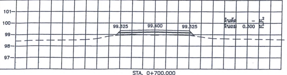
STA. 0+700.000 NGL = 98.944
