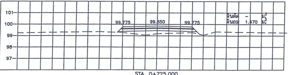
STA. 0+725.000 NGL = 99.174
