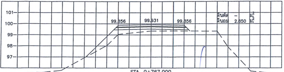
STA. 0+767.000 NGL = 99.356
