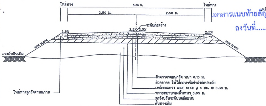
รูปตัดแนวดิ่ง โครงสร้างถนนคอนกรีตเสริมเหล็กและคลุมลัมบัติวัด
