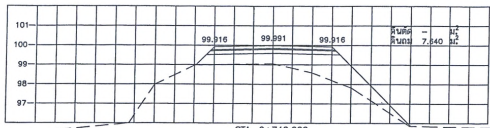
STA. 0+740.000 NGL = 99.056
