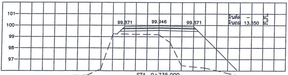
STA. 0+735.000 NGL = 99.174
