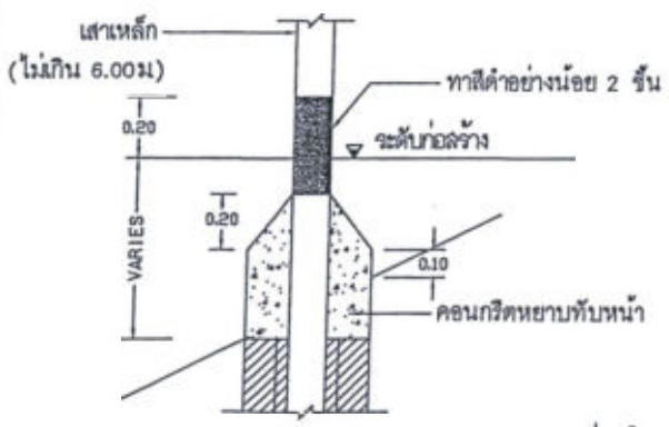
แสดงการปักเสาป้าย (ข้างซ้ายตลอดป้าย) และ (น-1)
