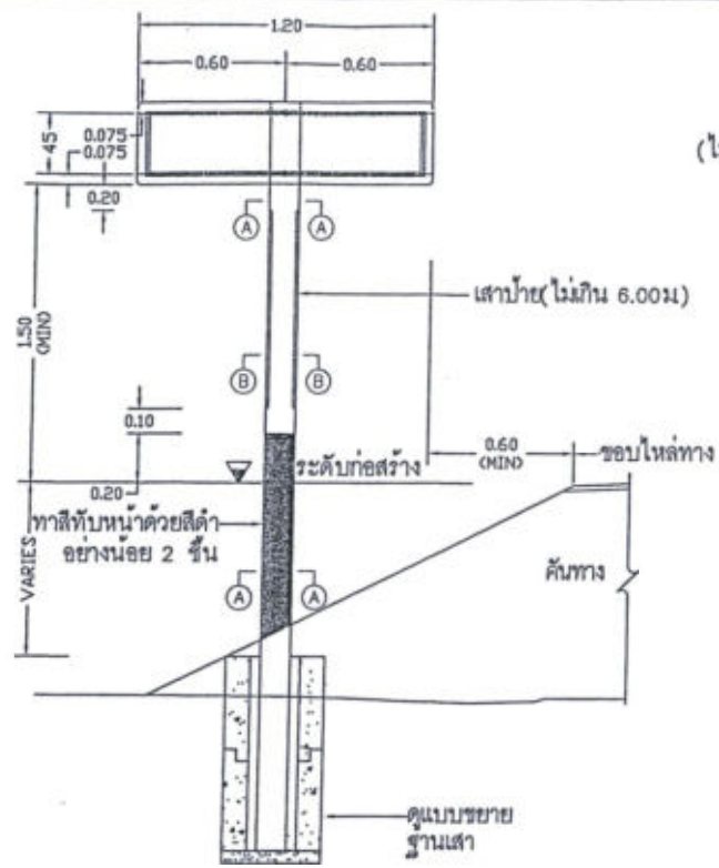
แสดงการปักเสาป้าย (ข้างซ้ายตลอดป้าย) และ (น-1)
