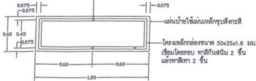
รายละเอียดด้านหลังป้าย (ขับขี่ปลอดภัย)
