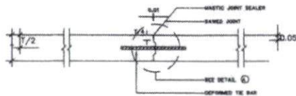
LONGITUDINAL JOINT
