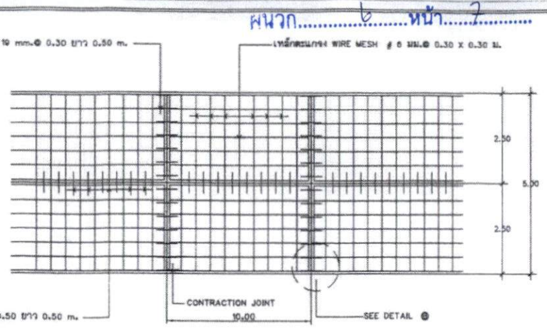
แปลนแนวดิ่งการเสริมเหล็กถนน ค.ล.ล.
