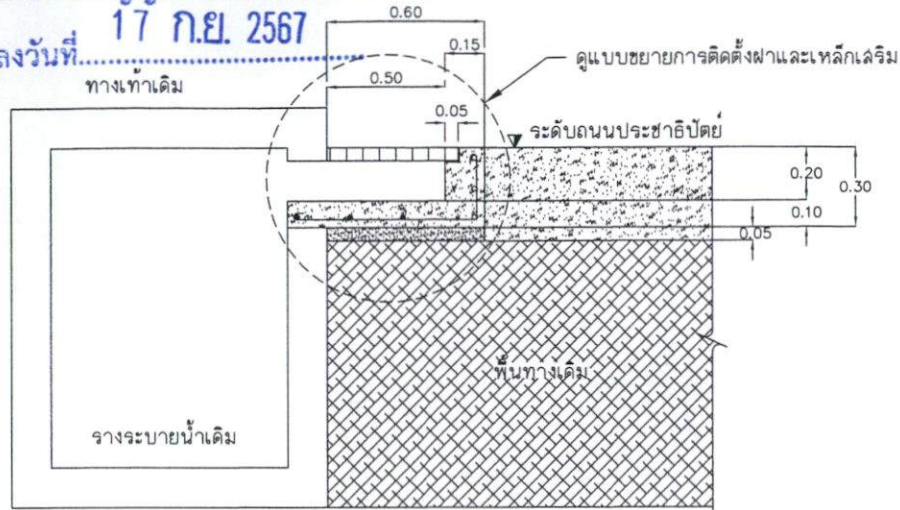
รูปตัดขยายการติดตั้ง
