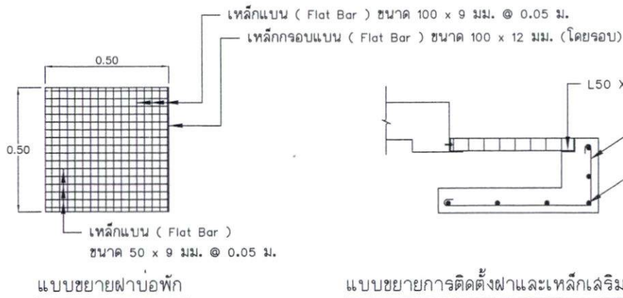
รูปตัดขยายการติดตั้ง
