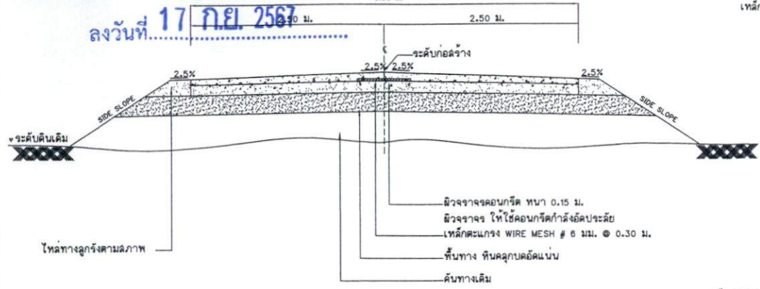
รูปตัดแสดงโครงสร้างถนนคอนกรีตเสริมเหล็กและคลุมมบัติวาลคู่
