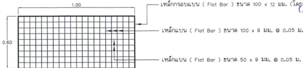
แบบขยายฝ้าปิดรางระบายน้ำ
