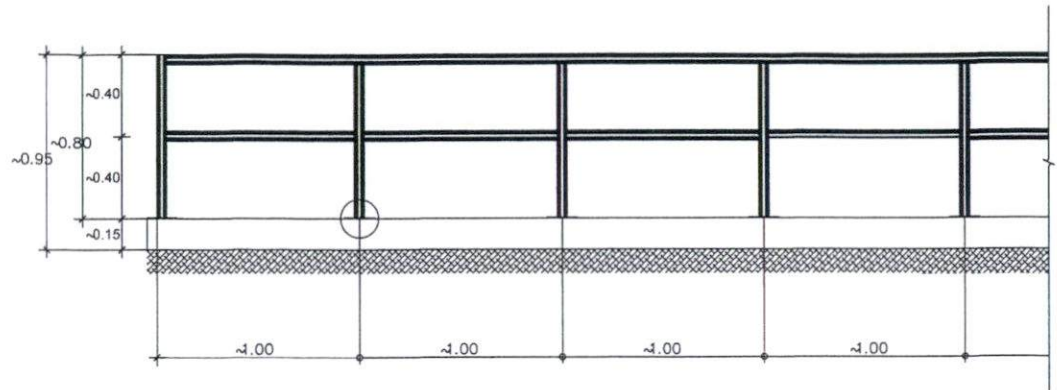
งานติดตั้งราวกันตกเหล็กรูปพรรณ
