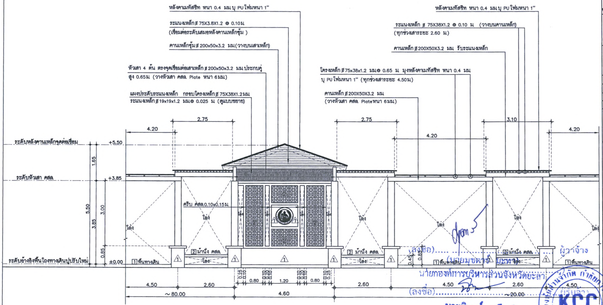
รูปด้าน 3 ขุมทางเดิน (1A) 1 : 75
