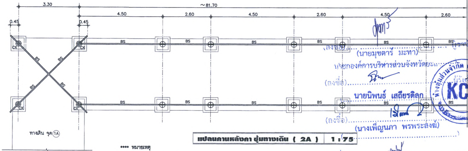
แปลนหลังคา-แนวเหล็กขุมทางเดิน ( 2A ) 1 : 75
