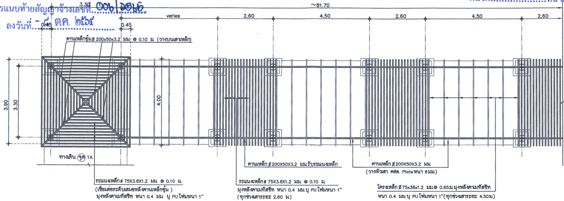
แปลนหลังคา-แนวเหล็กขุมทางเดิน ( 2A ) 1 : 75
