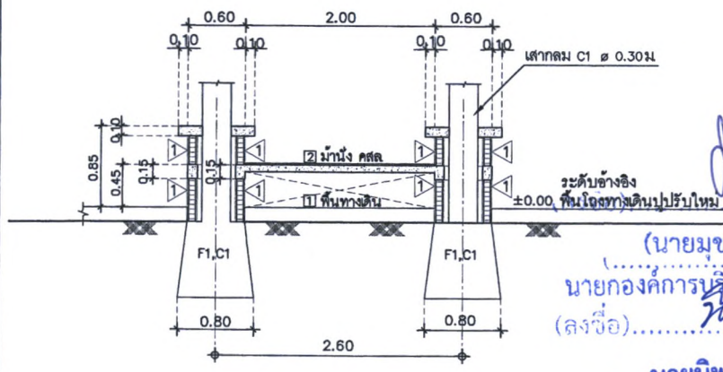
รูปตัด 1 1:50
