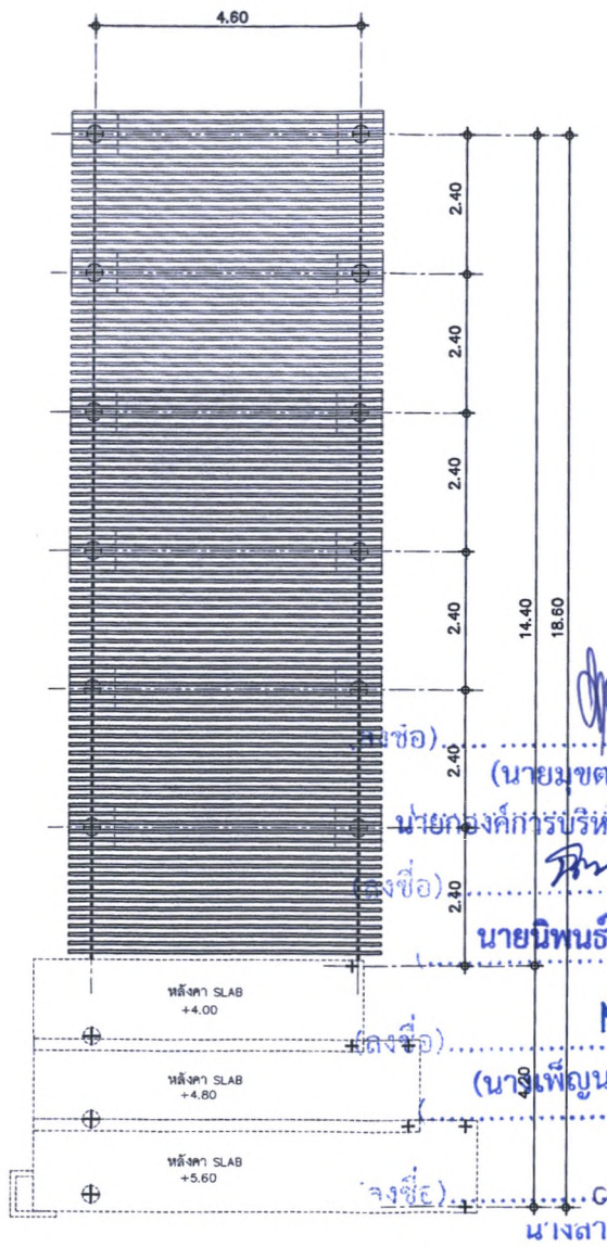
แปลนหลังคาแบบเหล็ก ( ชั้นทางเข้า ของเดิม ) 1 : 100
