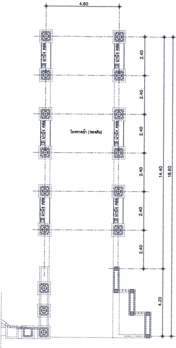
แปลนพื้น ( ชั้นทางเข้า ของเดิม ) 1 : 100
