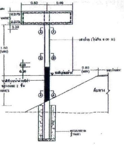
แสดงการปักเสาป้ายโครงการ ไม่แสดงราคาส่วน
