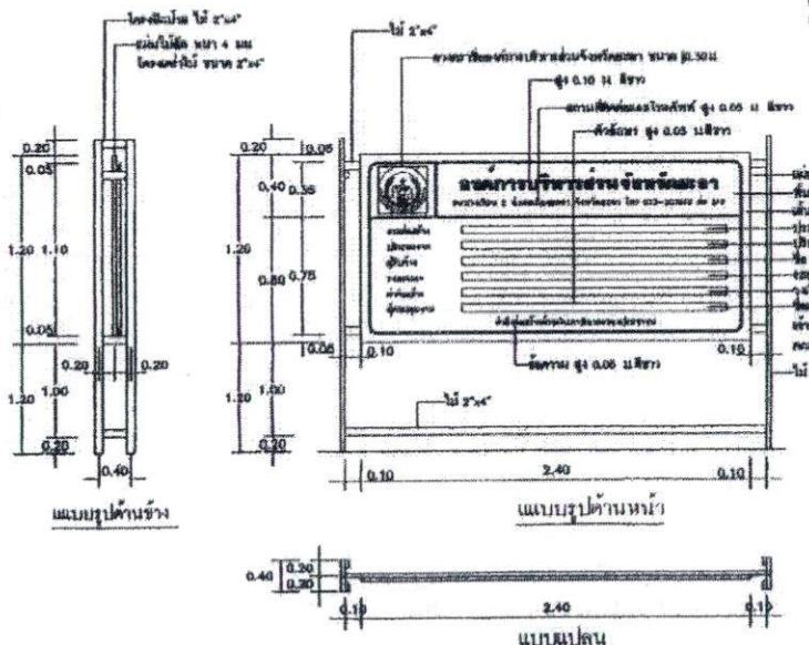
แนบป้ายแสดงรายละเอียดงานก่อสร้างขนาดเล็ก (ก.2) ขนาด 1.20x2.40 ม ไม่แสดงราคาส่วน
