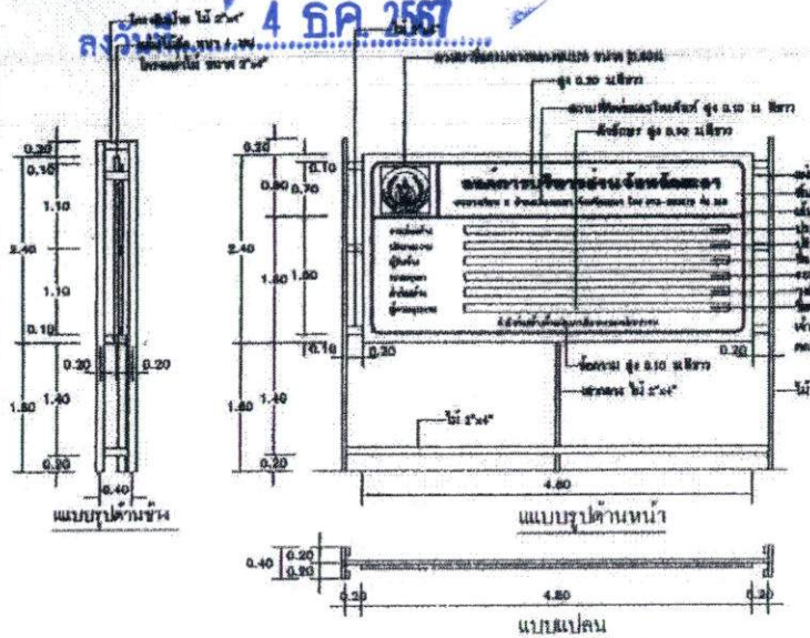
แนบป้ายแสดงรายละเอียดงานก่อสร้างขนาดใหญ่ (ก.1) ขนาด 2.40x4.80 ม ไม่แสดงราคาส่วน
