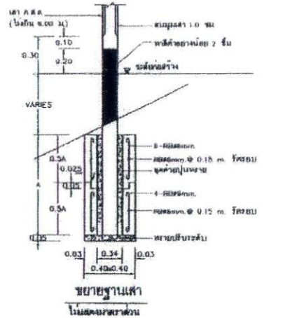
แสดงการปักเสาป้ายโครงการ ไม่แสดงราคาส่วน
