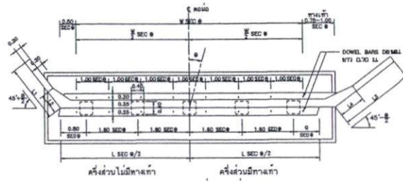
ครึ่งส่วนไม่มีทางท่า ครึ่งส่วนมีทางท่า แสดงแปลนคอกงอฐานแผ่ มาตราส่วนแบบที่ 1
