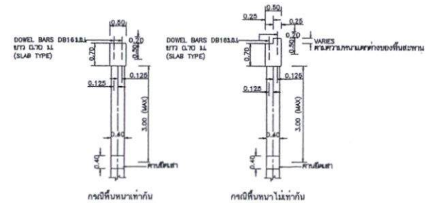
รูปตัด ๑ ๑ แสดงสัดส่วน
