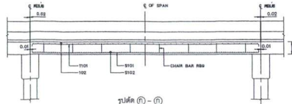
รูปตัด (ก) - (ก)
