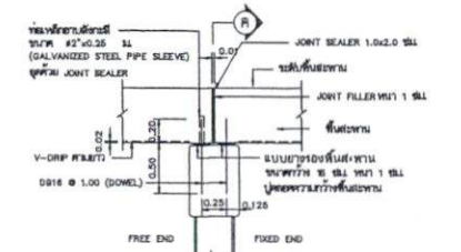
แสดงรายละเอียดหน้าตัด
