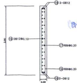
แสดงรูปตัด (๕) - (๕) มาตราส่วนแบบที่ 2
