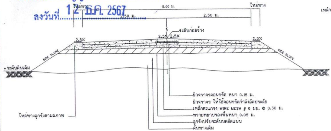
รูปตัดแฉ่งโครงสร้างถนนคอนกรีตเสริมเหล็กและคุณสมบัติวัสดุ
