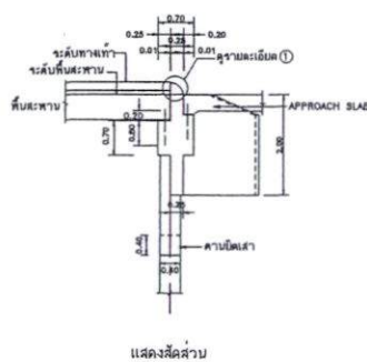
แสดงรูปตัด (๕) - (๕) มาตราส่วนแบบที่ 1
