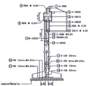
แสดงตัดคอกงอฐานแผ่
