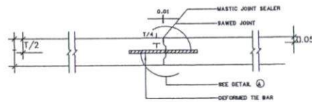
LONGITUDINAL JOINT
