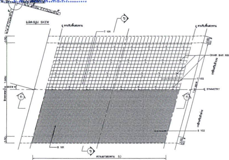
แผนผังแสดงการเสริมเหล็กที่หน้าตัด
