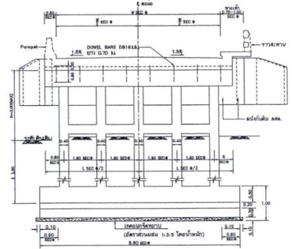
ครึ่งส่วนไม่มีทางท่า ครึ่งส่วนมีทางท่า แสดงตัดคอกงอฐานแผ่ มาตราส่วนแบบที่ 1
