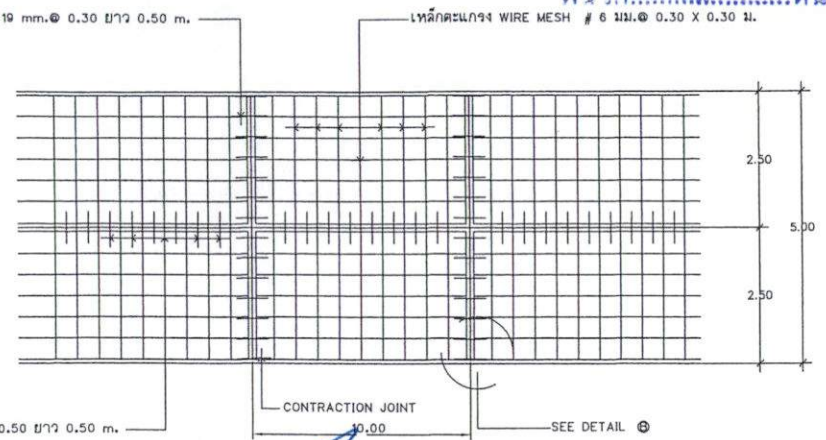
แผนผังการเสริมเหล็กถนน ค.ล.ล.
