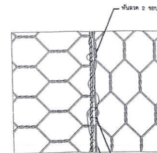
รูปที่ 1.2 วิธีการผูกกล่องลวดตาข่าย
