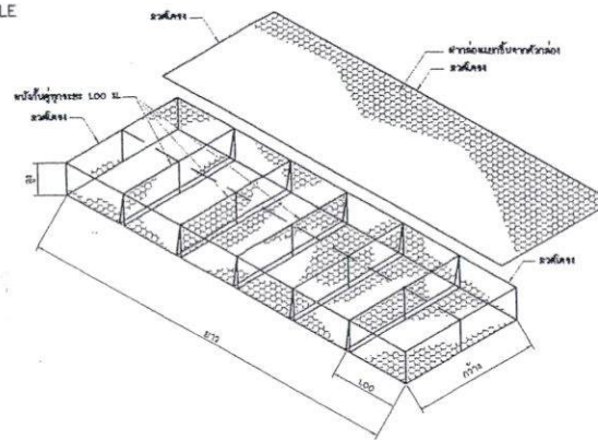
หมายเหตุ เส้นประหมายถึงส่วนที่ไม่มีลวดโครง (ข) ลักษณะทั่วไปของกล่องลวดตาข่ายแบบทแยง
