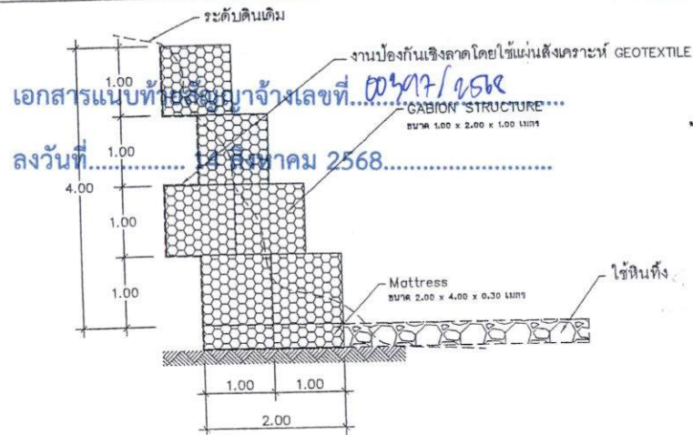
รูปตัดโครงสร้างป้องกันตลิ่ง
