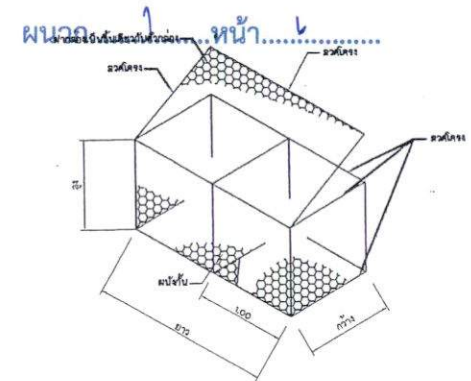
(หมายเหตุ เส้นประหมายถึงส่วนที่ไม่มีลวดโครง) (ก) ลักษณะทั่วไปของกล่องลวดตาข่ายแบบตรง
