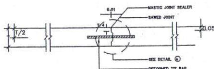
LONGITUDINAL JOINT
