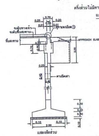
รูปตัด ๕-๕ มาตราส่วนแบบที่ 1
