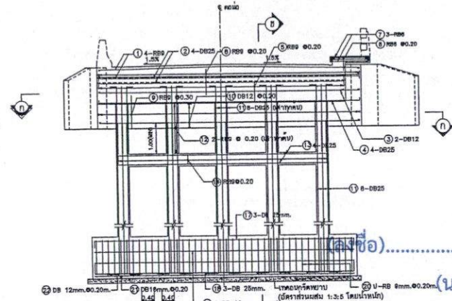
แสดงรูปตัด ๑-๑ มาตราส่วนแบบที่ 1
