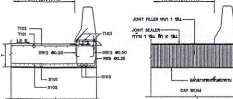
รูปตัด (ก) - (ค) แสดงรอยต่อที่ขึ้นสะพาน รูปตัด (ข) - (ง) แสดงรอยต่อที่ขึ้นสะพาน
