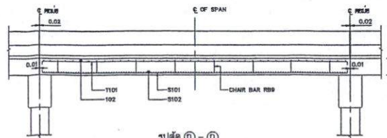
รูปตัด ก - ก มาตราส่วนย่อ 4
