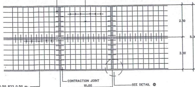
แปดนแสดงการเล่ริมเหล็กถนน ค.ล.ล.
