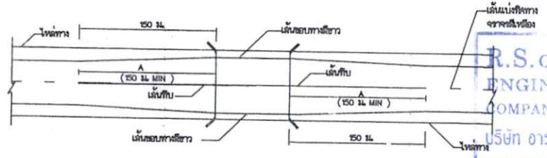
การตีเส้นจราจรที่มีความกว้างสะพานมากกว่าความกว้างผิวจราจรถนน ไม่แสดงมาตราส่วน
