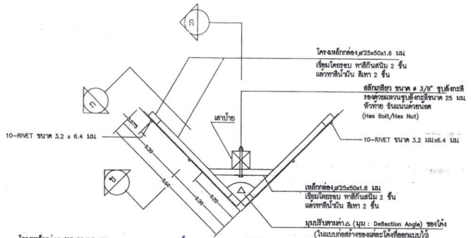
แปลนแสดงการติดตั้งป้าย ไม่แสดงขนาดส่วน
