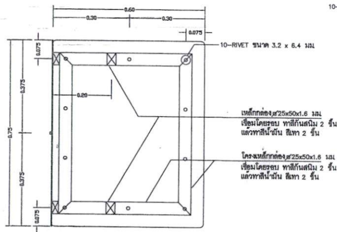
รูปด้าน ก การติดตั้งป้าย ไม่แสดงขนาดส่วน
