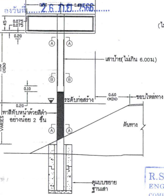
แสดงการปักเสาป้าย (ข้างซ้ายตลอดภัย) และ (น-1)
