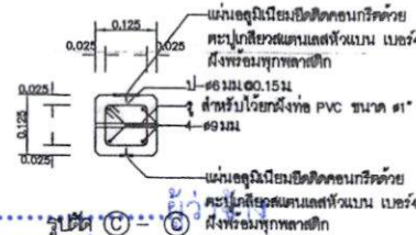
รูปตัด (B-B) ไม่แสดงมาตราส่วน
