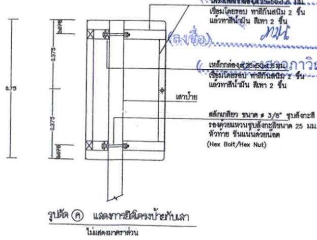
รูปตัด ๑) แสดงการติดตั้งป้าย ไม่แสดงขนาดส่วน
