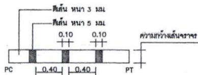
ขยาย 1 (ดูรายการประกอบแบบข้อ ๑)
