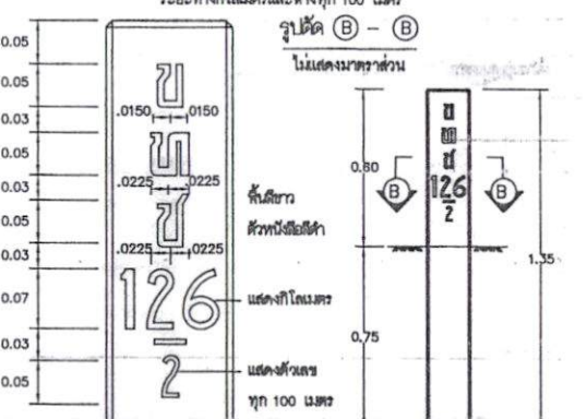
หลักเขตทาง ไม่แสดงมาตราส่วน
