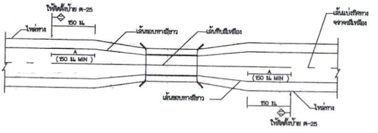
การตีเส้นจราจรที่มีความกว้างสะพานน้อยกว่าความกว้างผิวจราจรถนน ไม่แสดงมาตราส่วน
